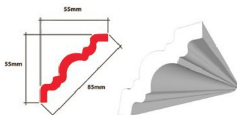
SANTE 55 x 55 x 85mm
